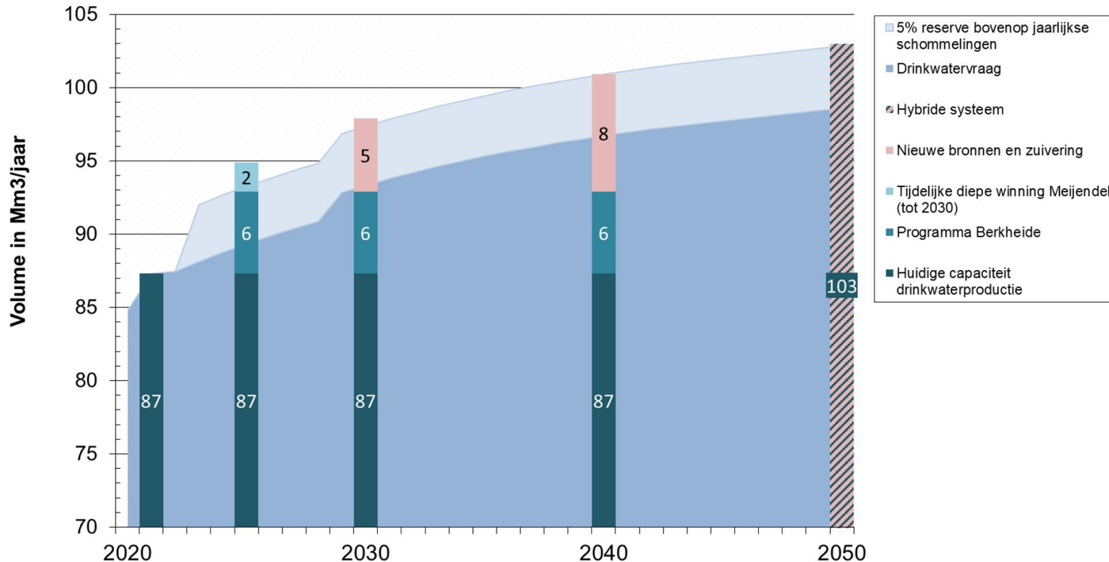
Drinkwaterproductie 2021-2050
